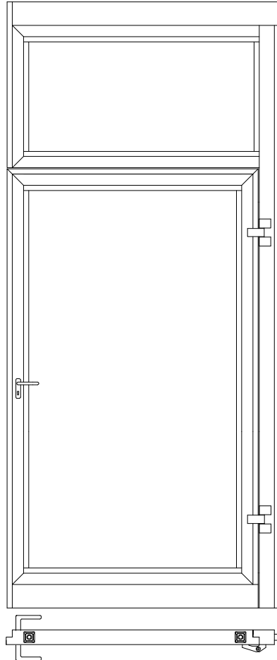
verfahrbares Schlupftürelement
